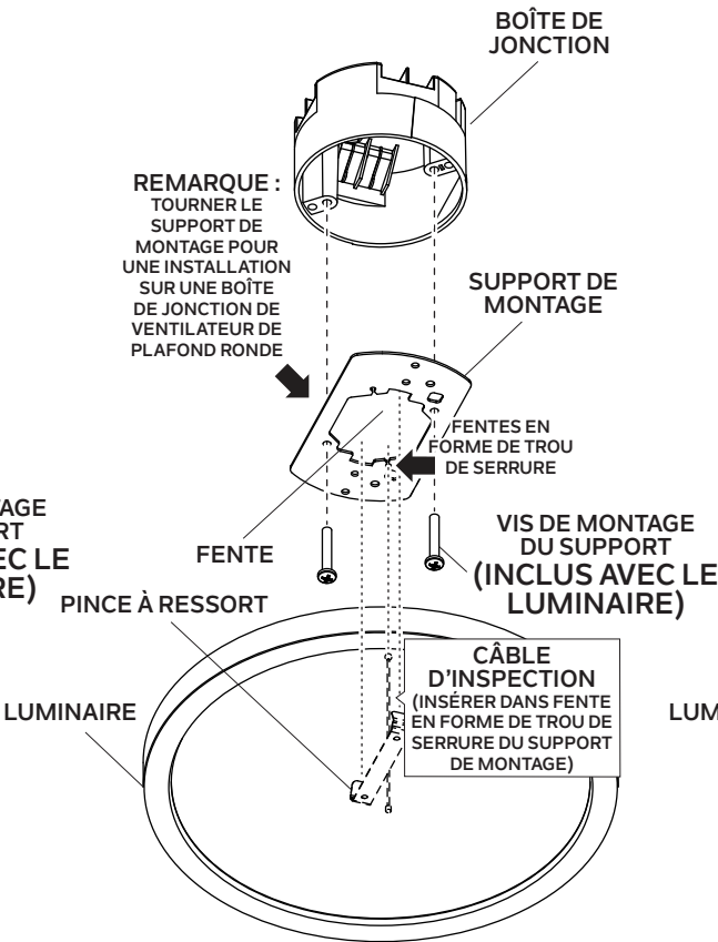
Fig. 2 INSTALLATION SUR LA BOÎTE DE JONCTION DU VENTILATEUR DE PLAFOND RONDE
