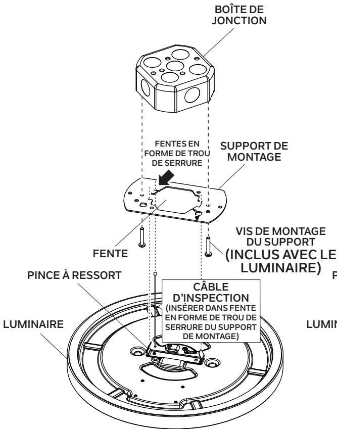
Fig. 1 INSTALLATION SUR UNE BOÎTE DE JONCTION STANDARD
